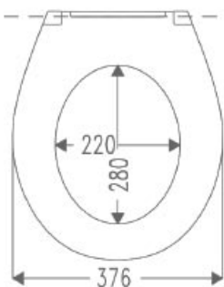
Maßzeichnung
